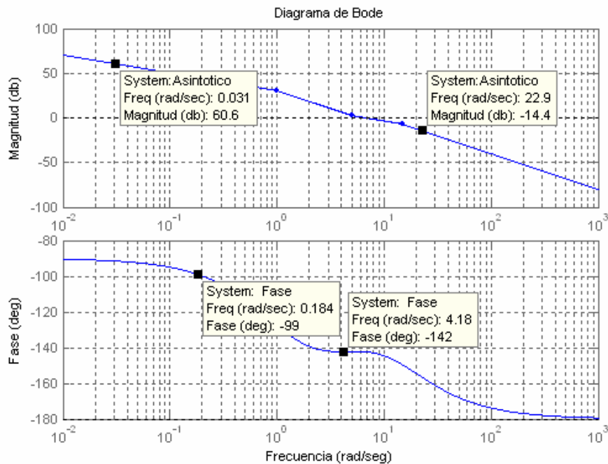
Figura 3. 12: Diagrama de Bode obtenido usando la función nbody.m
