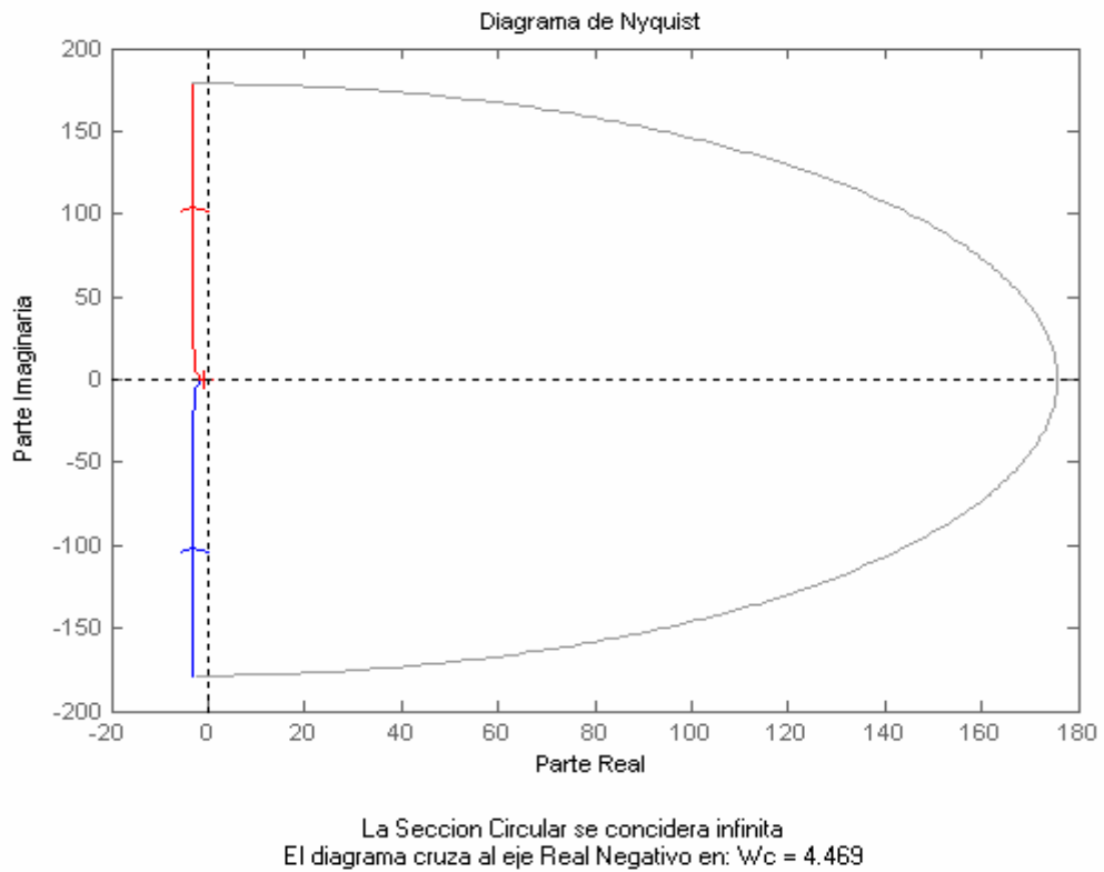
Figura 3. 2: Diagrama de Nyquist de G(s) usando la función mnyquist.m
