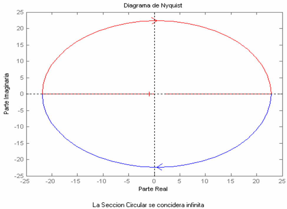
Figura 3. 7:Diagrama de Nyquist del ejemplo 3.1.3 usando la función mnyquist.m
